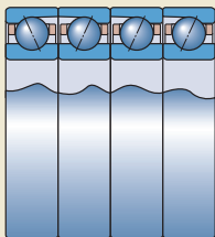
面对面+串联配置 代号后缀QFT
