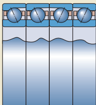
串联后面对面配置 代号后缀QFC
