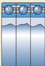
面对面+串联配置 代号后缀TFT
