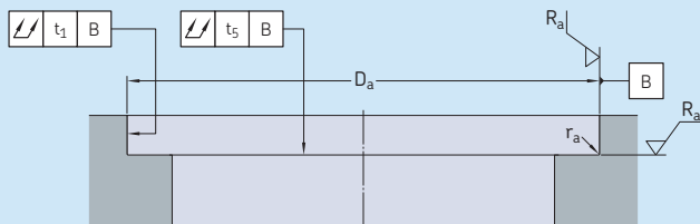
轴承座安装面的几何精度
