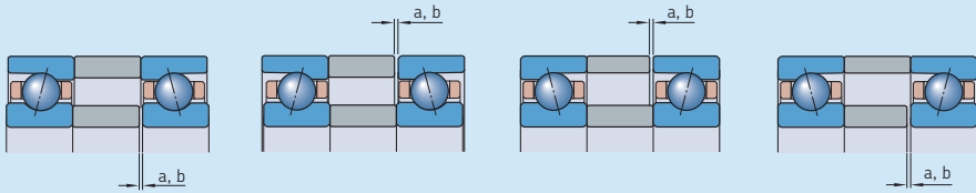
隔圈宽度减少量的指导值 - 718..D轴承系列
